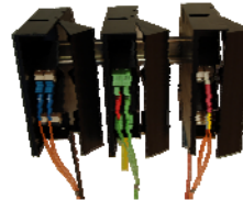
OPTOC4 4 x LC duplex oder 4 x SC/E-2000 30 x 130 x 127 mm (BxHxT)
